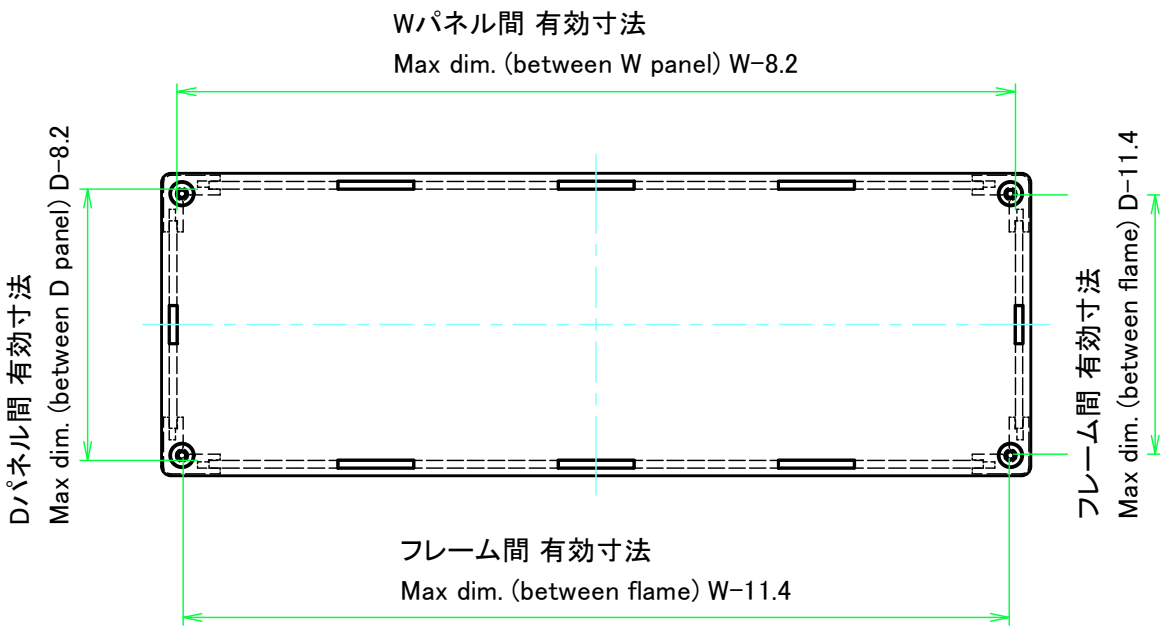
下カバー / Bottom cover
